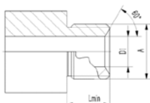
螺纹管路应用
