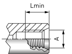
依据 SAE J514 JIC37 标准
