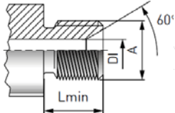
公制 ISO 螺纹管连接 依据 DIN 7631 / DIN 7647
