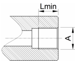
依据公制 ISO 螺纹
