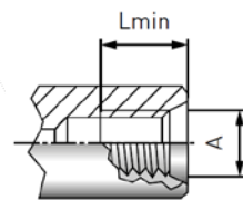
公制 ISO 螺纹 (DIN 13 – 根据 ISO 6149- 1)
