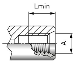
英制直管螺纹 依据 DIN ISO228-1 标准
