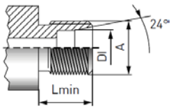
公制 ISO 螺纹管连接 依据 DIN 3902
