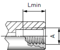
英制直管螺纹 依据 DIN ISO228-1
