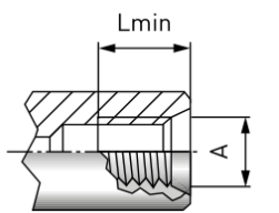
NPT-螺纹 (依据 ANSI/ASME B 1.20-1983 标准)
