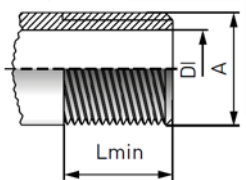
英制直管螺纹 依据 DIN ISO228-1 标准
