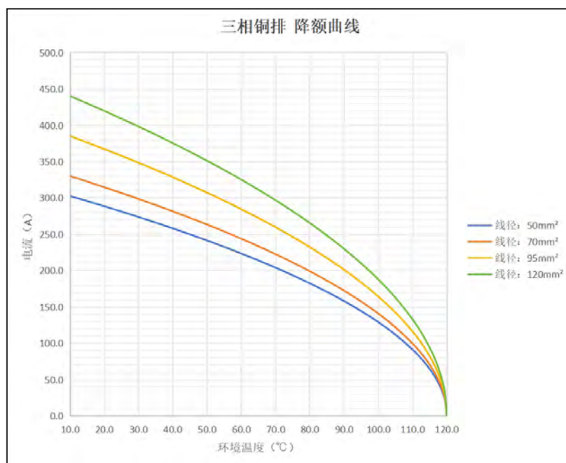
载流曲线
