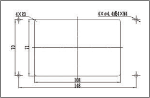
安装开孔图
