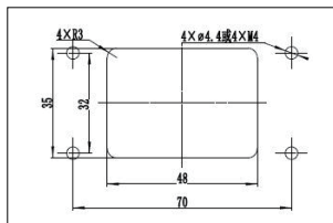
安装开孔图
