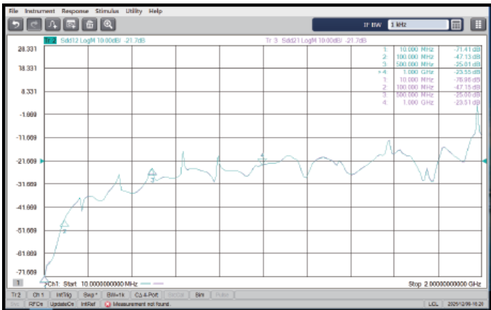
Sdd21/sdd12-NEXT 近端串扰（插拔5000次后）
