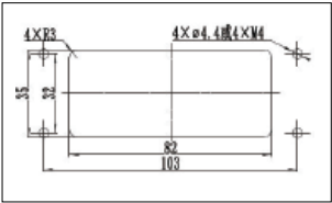
安装开孔图
