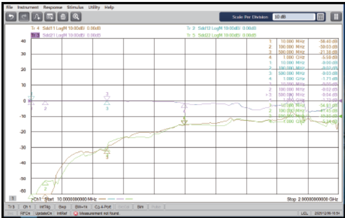
Sdd21/sdd12-插入损耗 sdd11/sdd22-回波损耗（未插拔）
