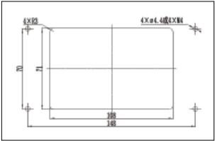
安装开孔图
