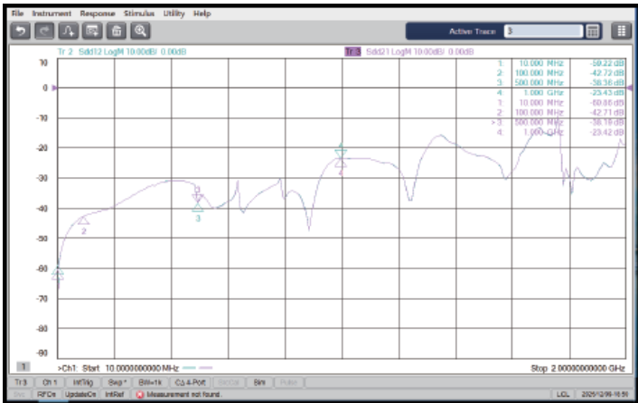
Sdd21/sdd12-NEXT 近端串扰（未插拔）
