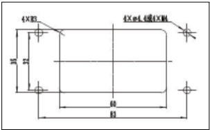
安装开孔图
