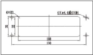
安装开孔图
