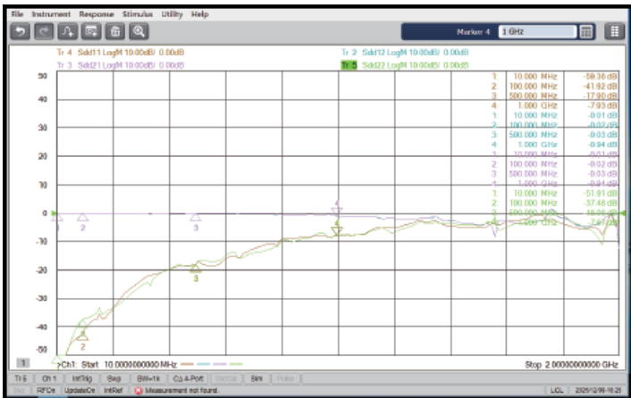
Sdd21/sdd12-插入损耗 sdd11/sdd22-回波损耗（插拔5000次后）
