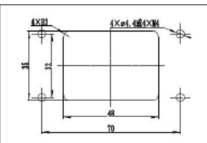
安装开孔图
